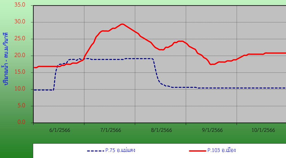
กราฟแสดงปริมาณน้ำปิ้งรายชั่วโมงรอบวันที่ 1/2566 ที่สถานีแม่ น้ำปิ้ง (P.75) บ้านซ้อแล อ.แม่แตง และที่สถานีแม่ น้ำปิ้ง(P.103) บ้านป่าซ่อยใต้ อ.เมือง จ.เชียงใหม่
